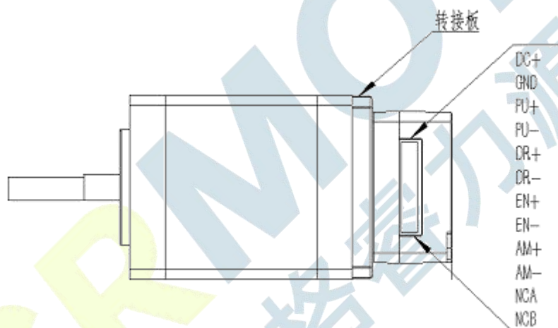
图 3.1 IDH35 接口示意图
